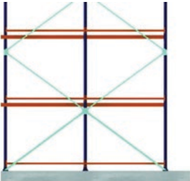
Düşey çapraz (Zemine bağlı) Vertical cross-bracings (Depending on floor type)
